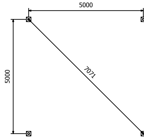
A-A Fundamentsplan
