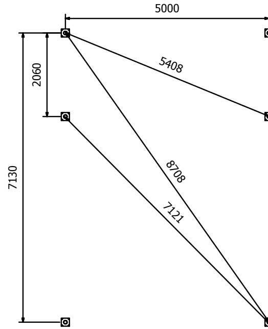
A-A Fundamentsplan
