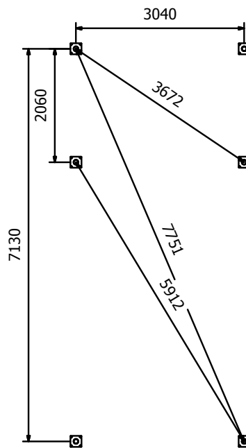
A-A Fundamentsplan
